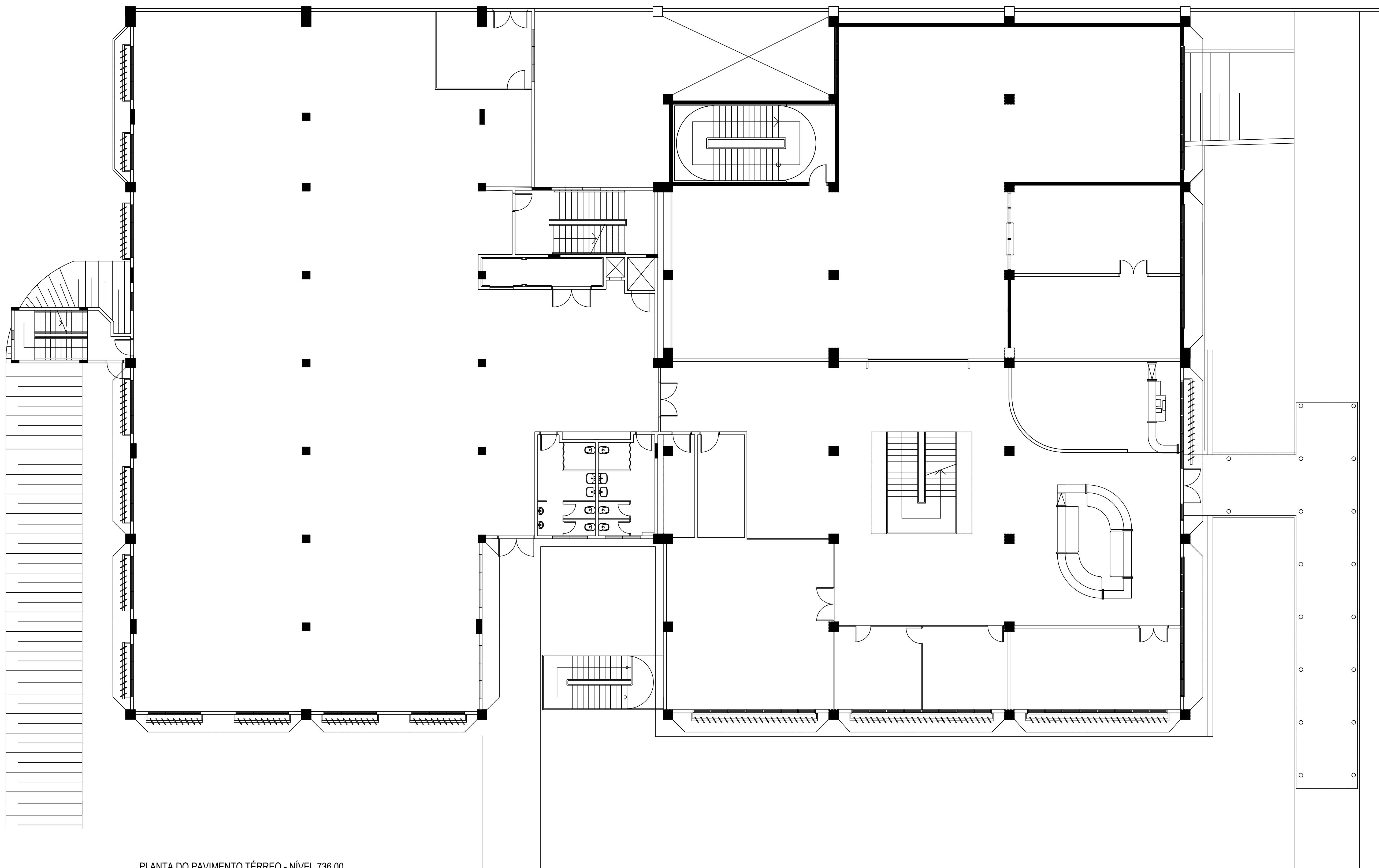
PLANTA DO PAVIMENTO TÉRREO - NÍVEL 736,00 ESCALA 1:100
